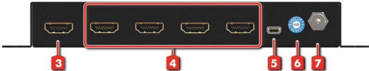
[図 3.2] リアパネルの外観図
