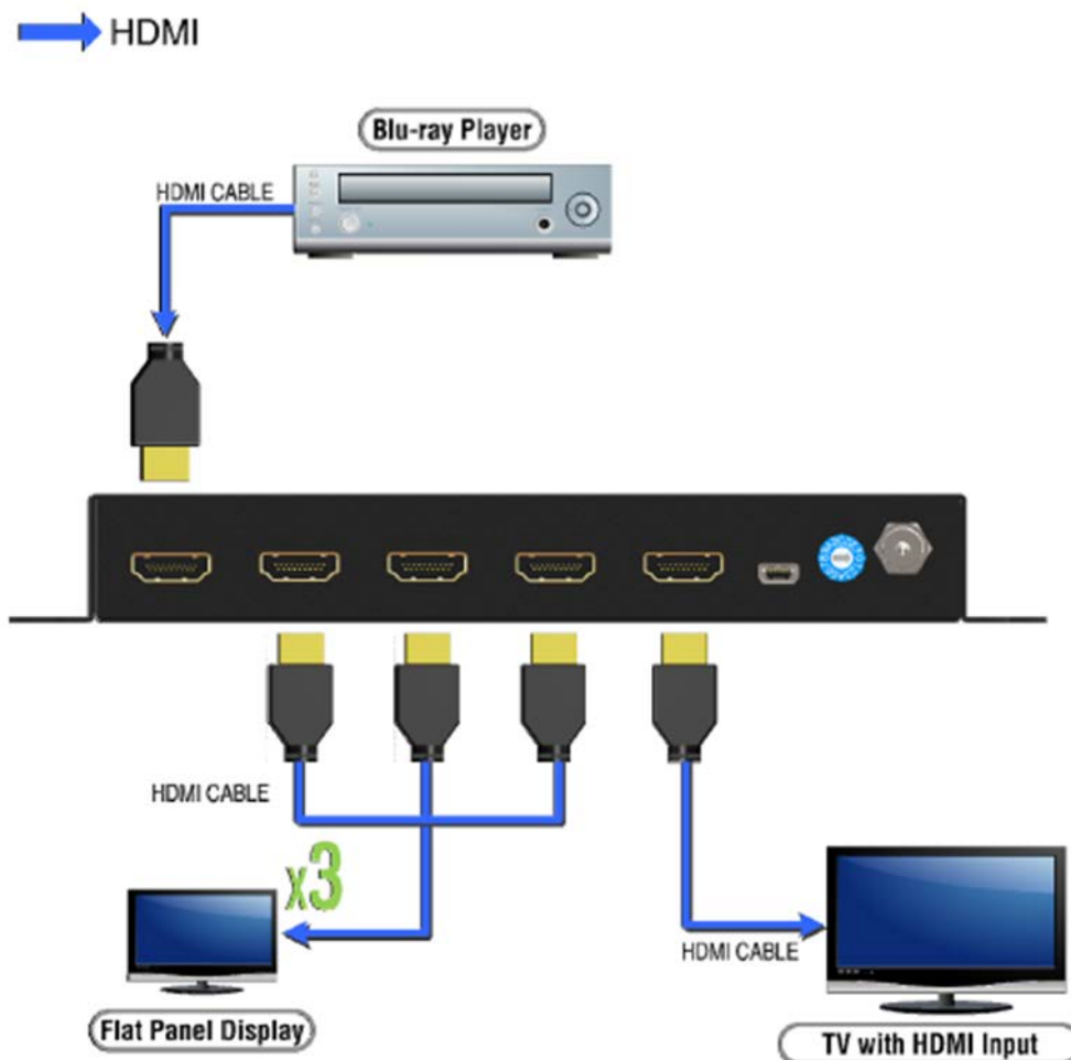
[図 4.1] ソース機器とシンク機器を接続したときの接続例
